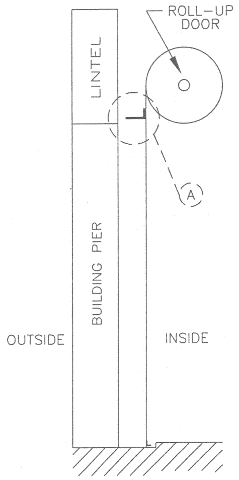
SECTION THRU DOOR N.T.S.
